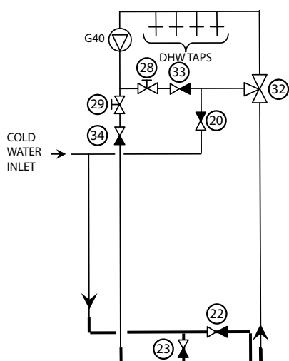
Bilde 1. Varmtvannssirkulasjon
