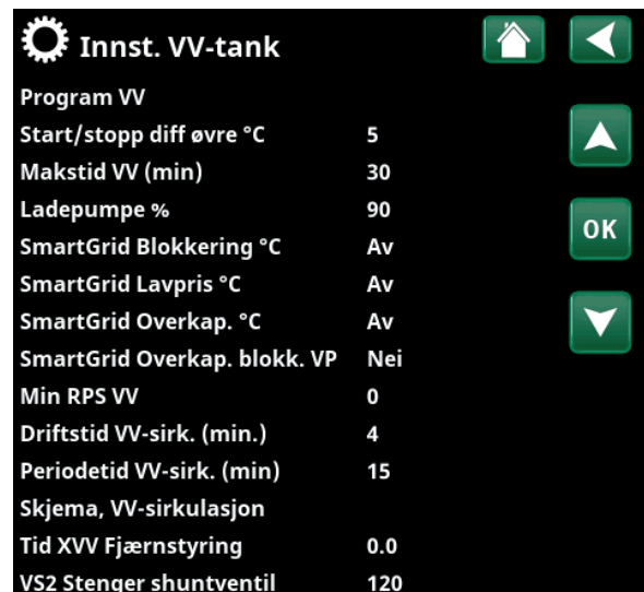
Meny «Avansert/Innstillinger/VV-tank».
