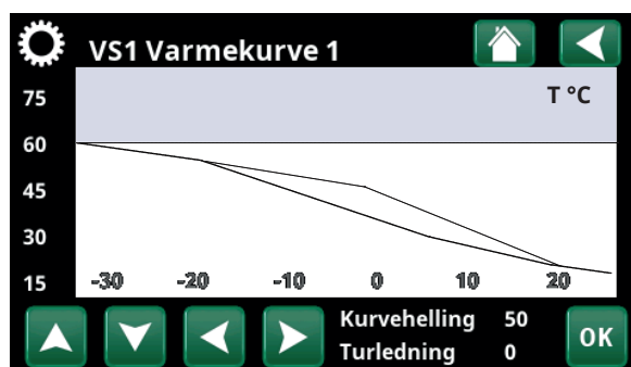
Meny «Avansert/Innstillinger/Varmesystem/Varmesystem1/Varmekurve».
