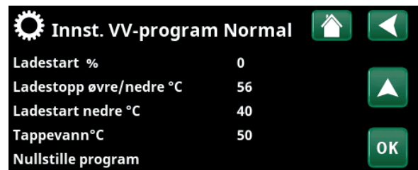
Menyen «Avansert/Innstillinger/Varmtvann/VV-program».
