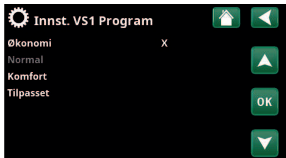
Meny «Avansert/Innstillinger/Varmesystem/Varmesystem1/Program».
