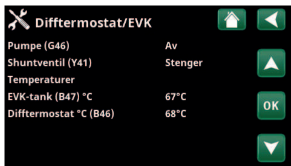
Meny «Avansert/Service/Funksjonstest/Difftermostat/EVK».
