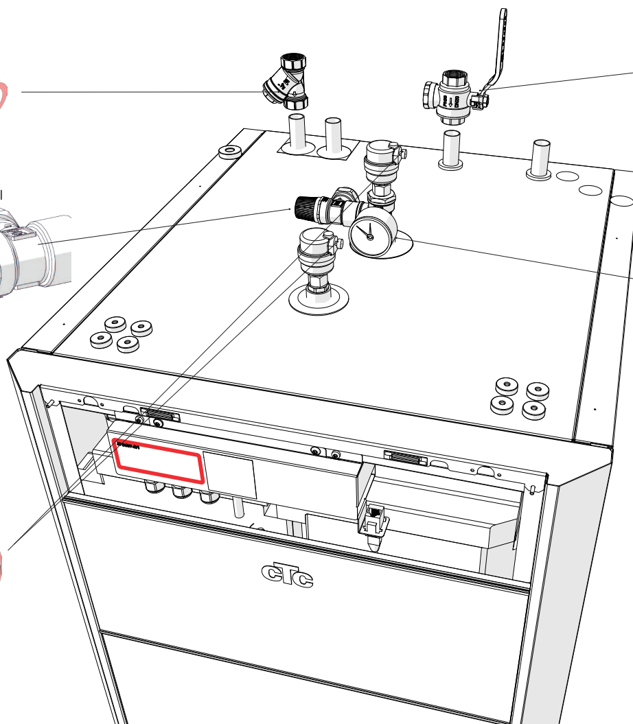
Sikkerhetsventil
