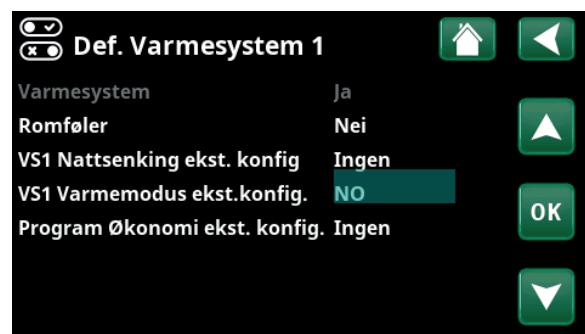
Meny «Avansert/Definere/Varmesystem/Varmesystem 1».
