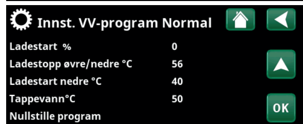
Menyen «Avansert/Innstillinger/Varmtvann/VV-program».
