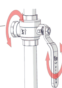
Magnetfilter kuleventil
