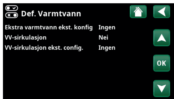
Menyen «Avansert/Definere/Varmtvann».
