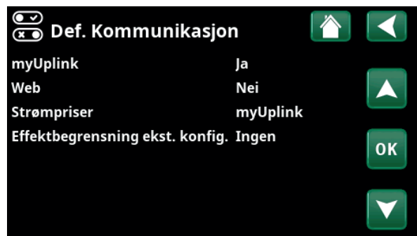
Meny «Avansert/Definere/Kommunikasjon».
