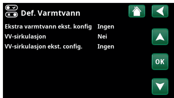
Menyen «Avansert/Definere/Varmtvann».
