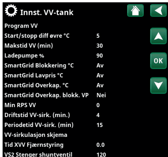
Meny «Avansert/Innstillinger/VV-tank».
