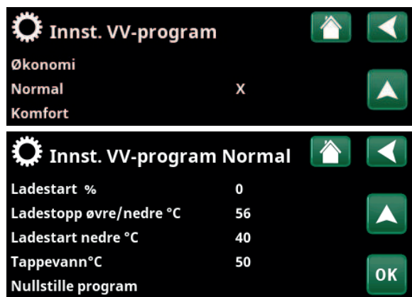
Menyen «Avansert/Innstillinger/Varmtvann/VV-program».
