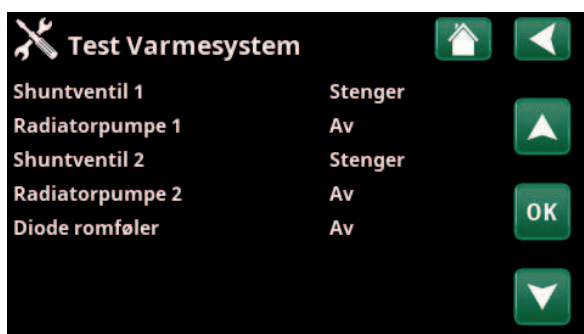
Meny «Avansert/Service/Funksjonstest/Varmesystem».
