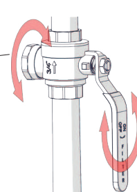
Magnetfilter kulventil
