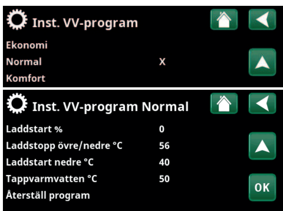
Menyer "Avancerat/Inställningar/Varmvatten/VV-program".
