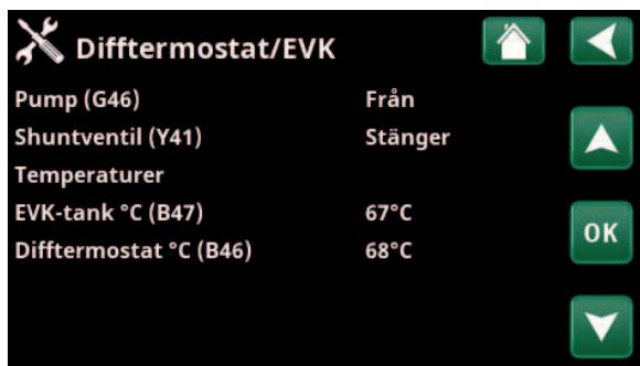
Meny "Avancerat/Service/Funktionstest/Difftermostat/EVK".
