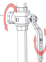
Magnetfilter kulventil
